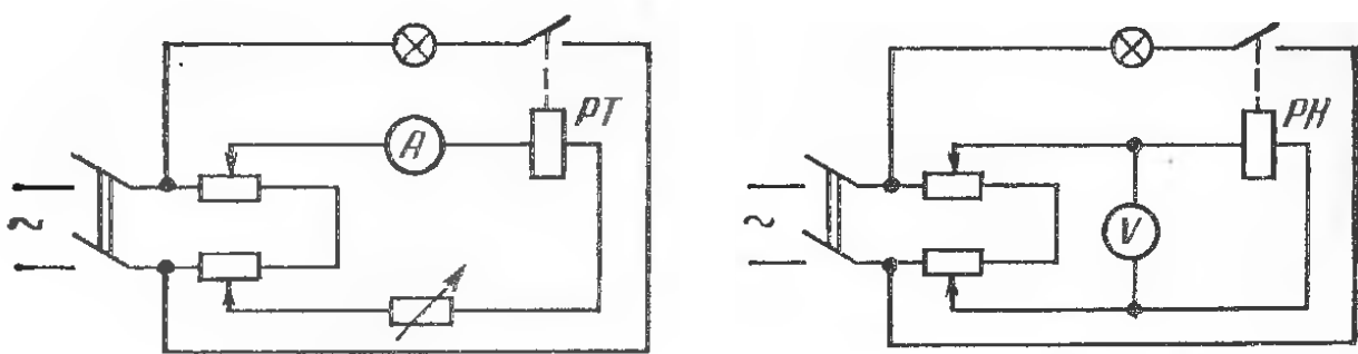
Рис. Схема испытаний реле тока (а) и реле напряжения (б)
